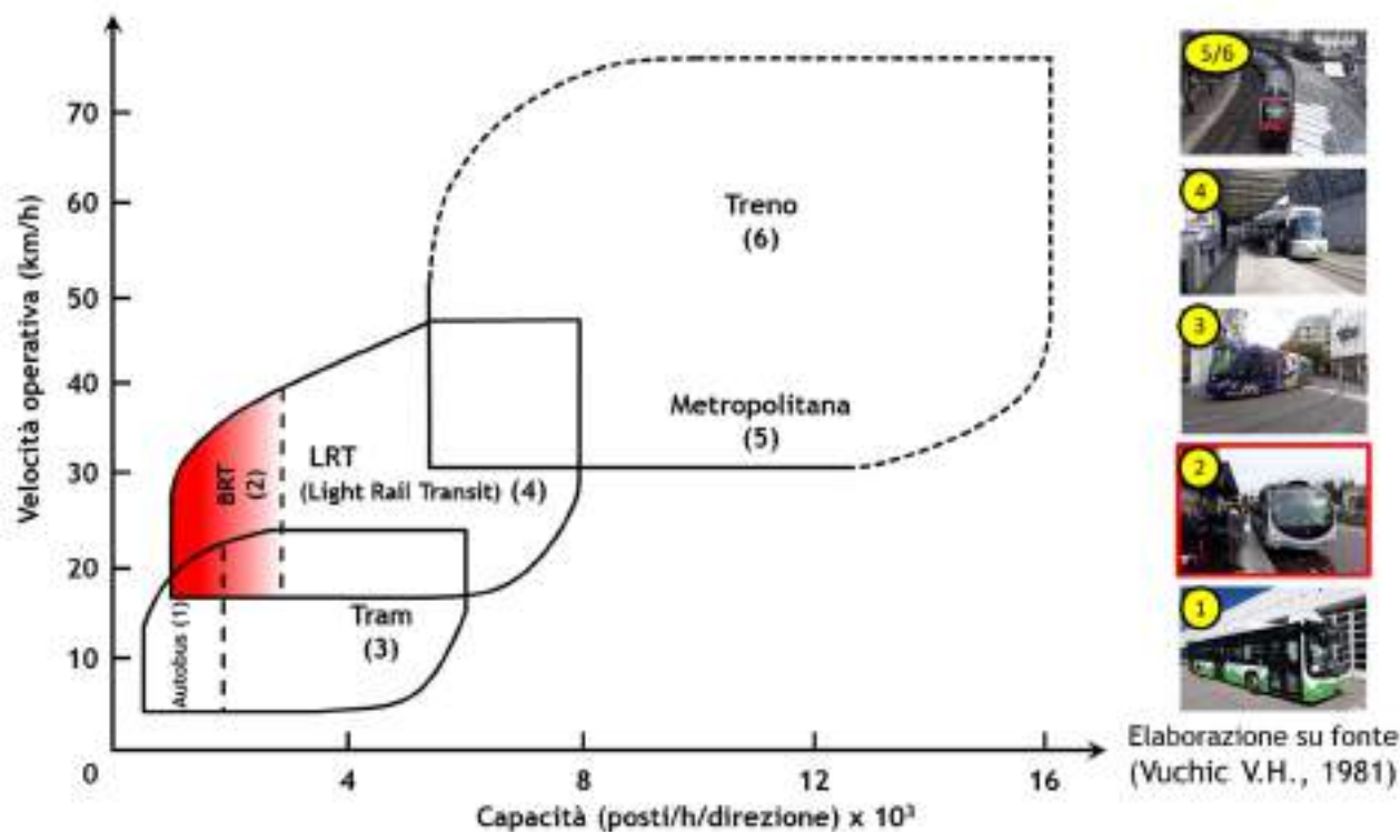
Figura 4-5 Specifiche tecniche dei sistemi BRT – Dominio ottimale di impiego. – elaborazioni TPS PRO su base da letteratura (Fonte: Vuchic V.H., 1981)
